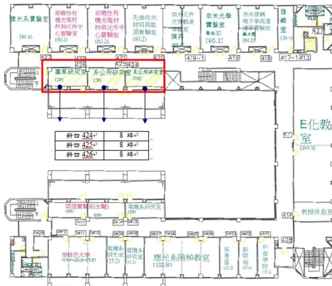
圖二、埔里園區育成實驗型培育室空間名稱與坪數圖
