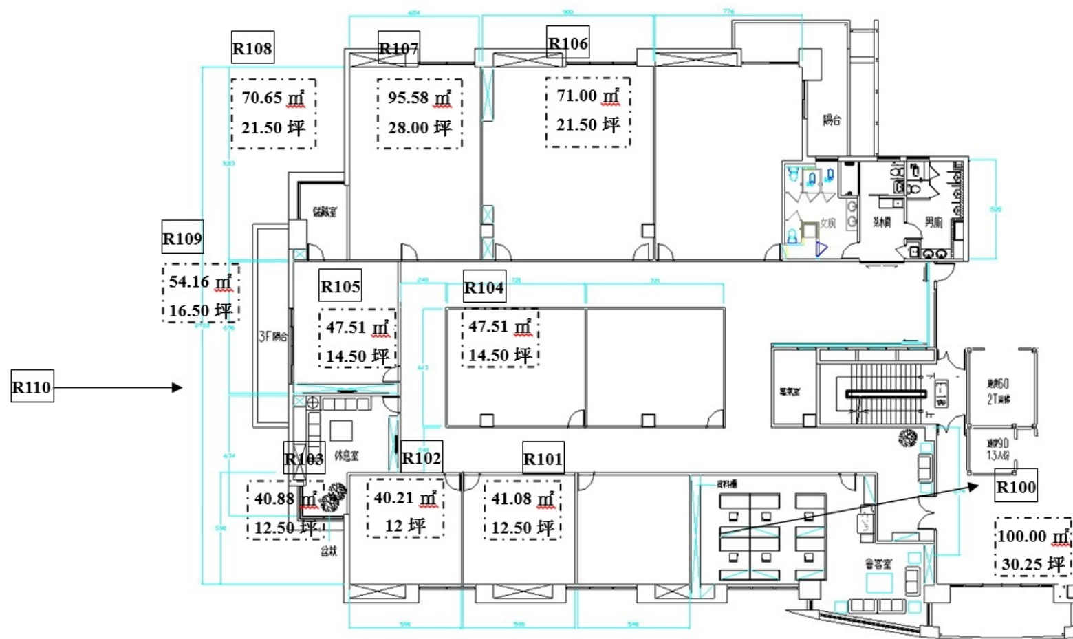
暨南大學創業育成中心平面配置圖 1:150
